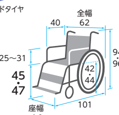
ハイブリッドタイヤ
