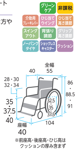
ウイング スイングアウト
