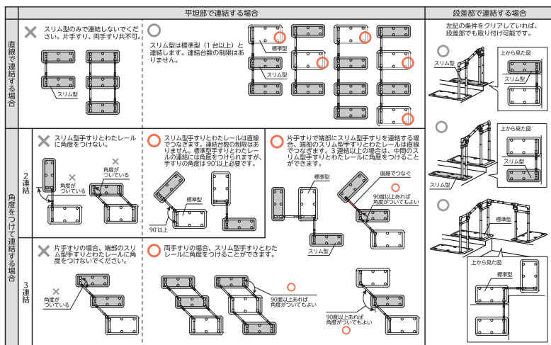
片手すり BZK-03S (N)
